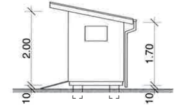
Stall Nagetiere - Ansicht Seite
