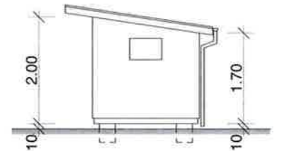
Stall Ziegen - Ansicht Seite
