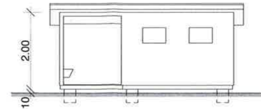
Stall Ziegen - Ansicht Front
